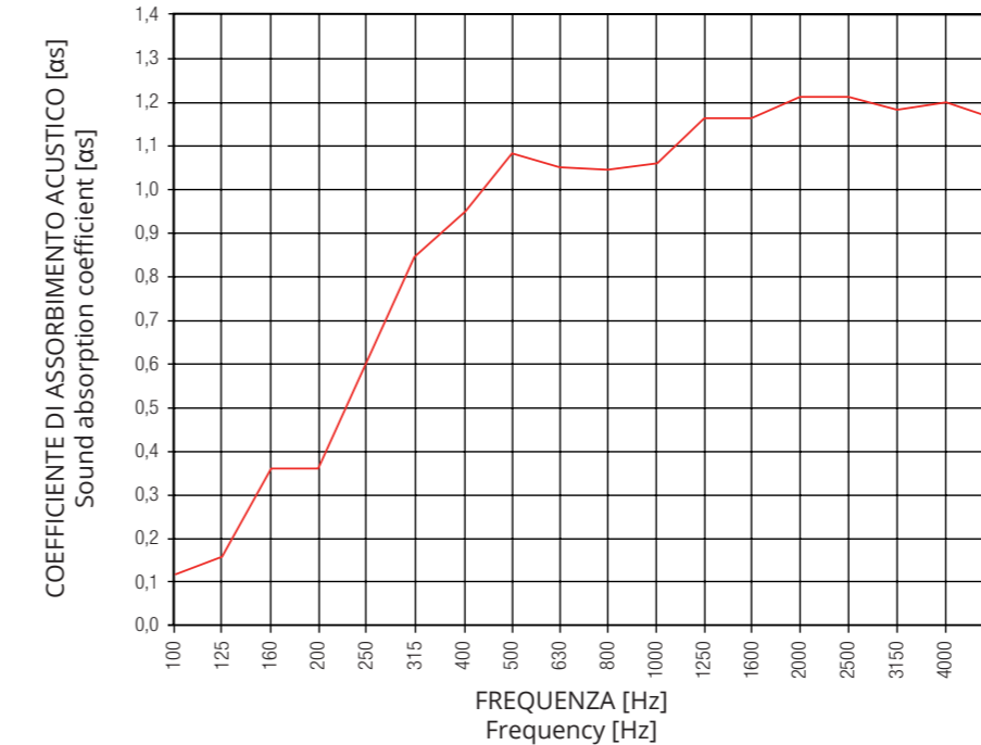
ANDAMENTO DEL COEFFICIENTE DI ASSORBIMENTO ACUSTICO "αs" PER TERZI D'OTTAVA One-third octave sound absorption coefficient curve "αs"
